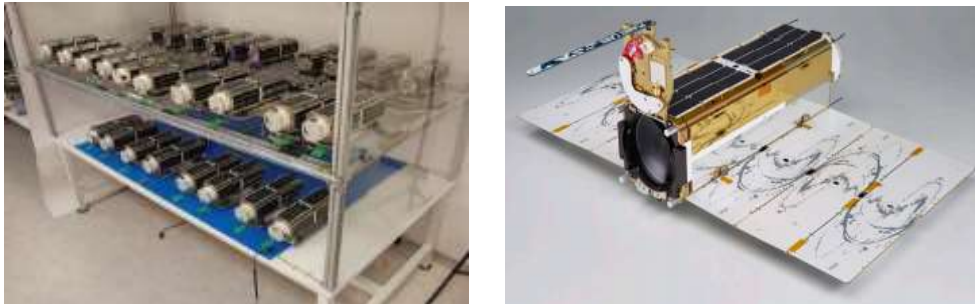
図表 18: Planet Labs 社が独自に開発する小型衛星「Dove」(上)と撮影画像(下)
