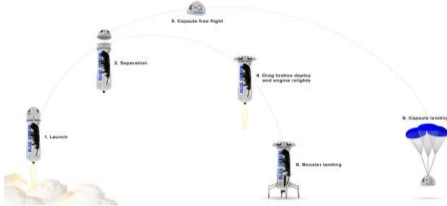
図表 13:「ニューシェパード」ロケットの垂直着陸の仕組み
